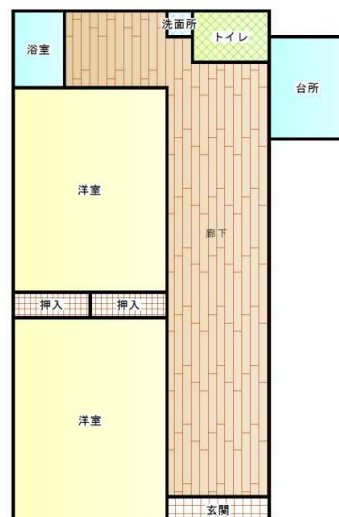
間取り
